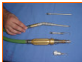
Ao lado, autoclave, abaixo, conjunto pneumático drill, trépano e craneótomo
